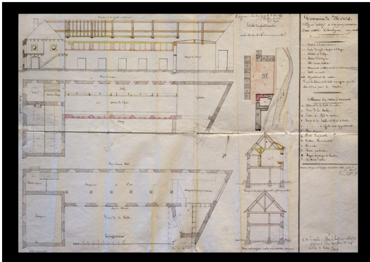
Commune de Morez. Projet relatif à l'appropriation d'un atelier d'horlogerie en petit [plans et coupes], 1854.
