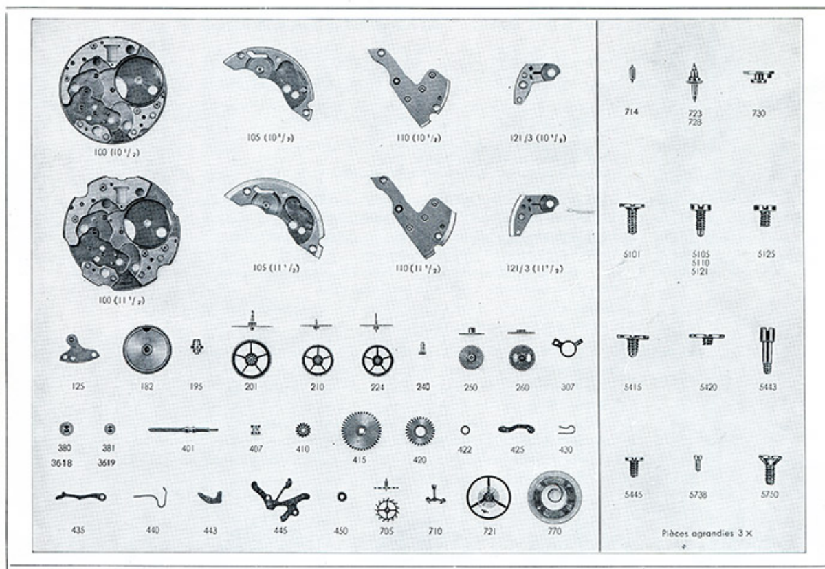
Calibre 10 1/2 - 11 1/2''' - 233-68 - fournitures du calibre de base, 1973.
