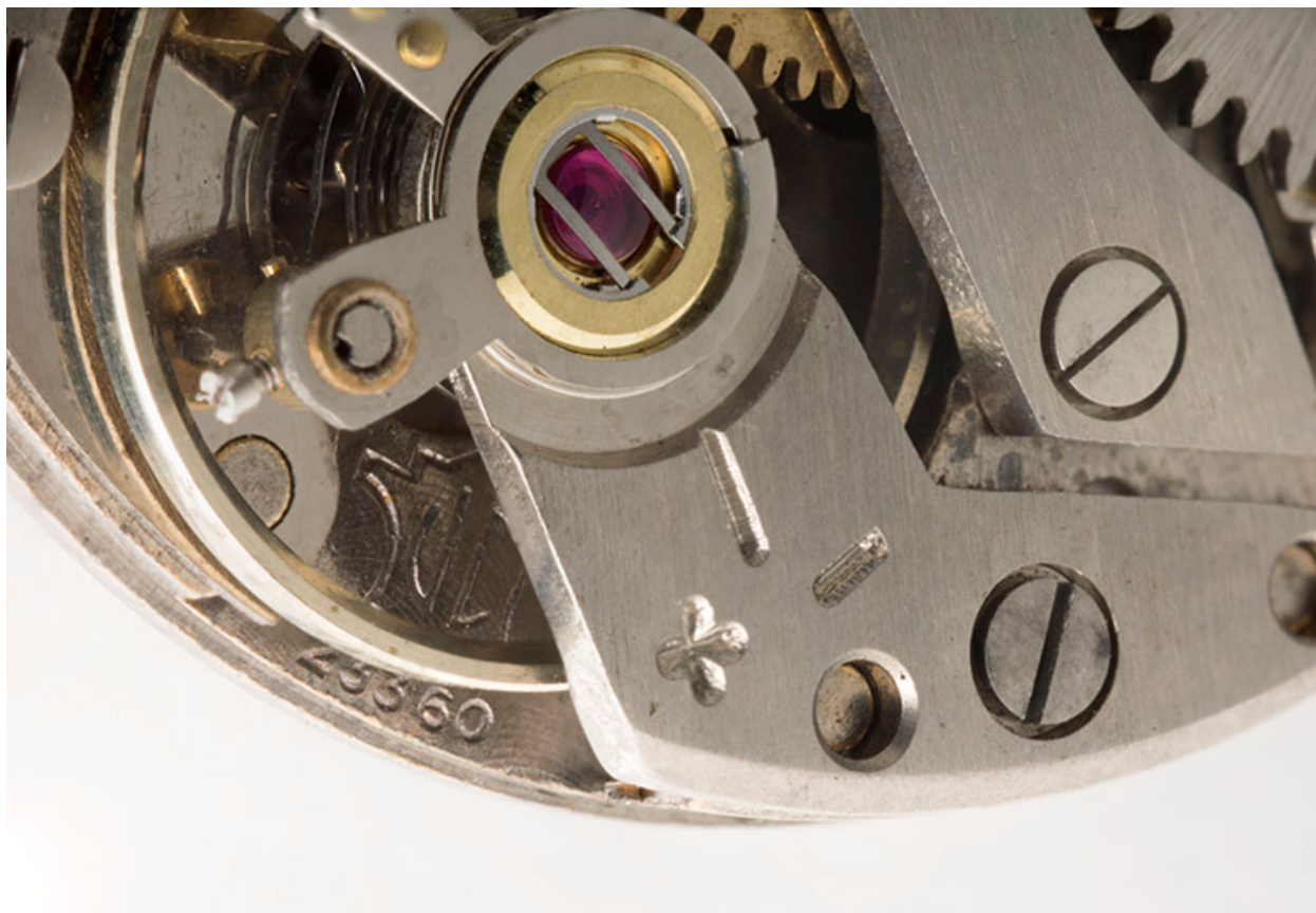
Mouvement Cupillard 233-60 : logotype de la société et indication du modèle.
