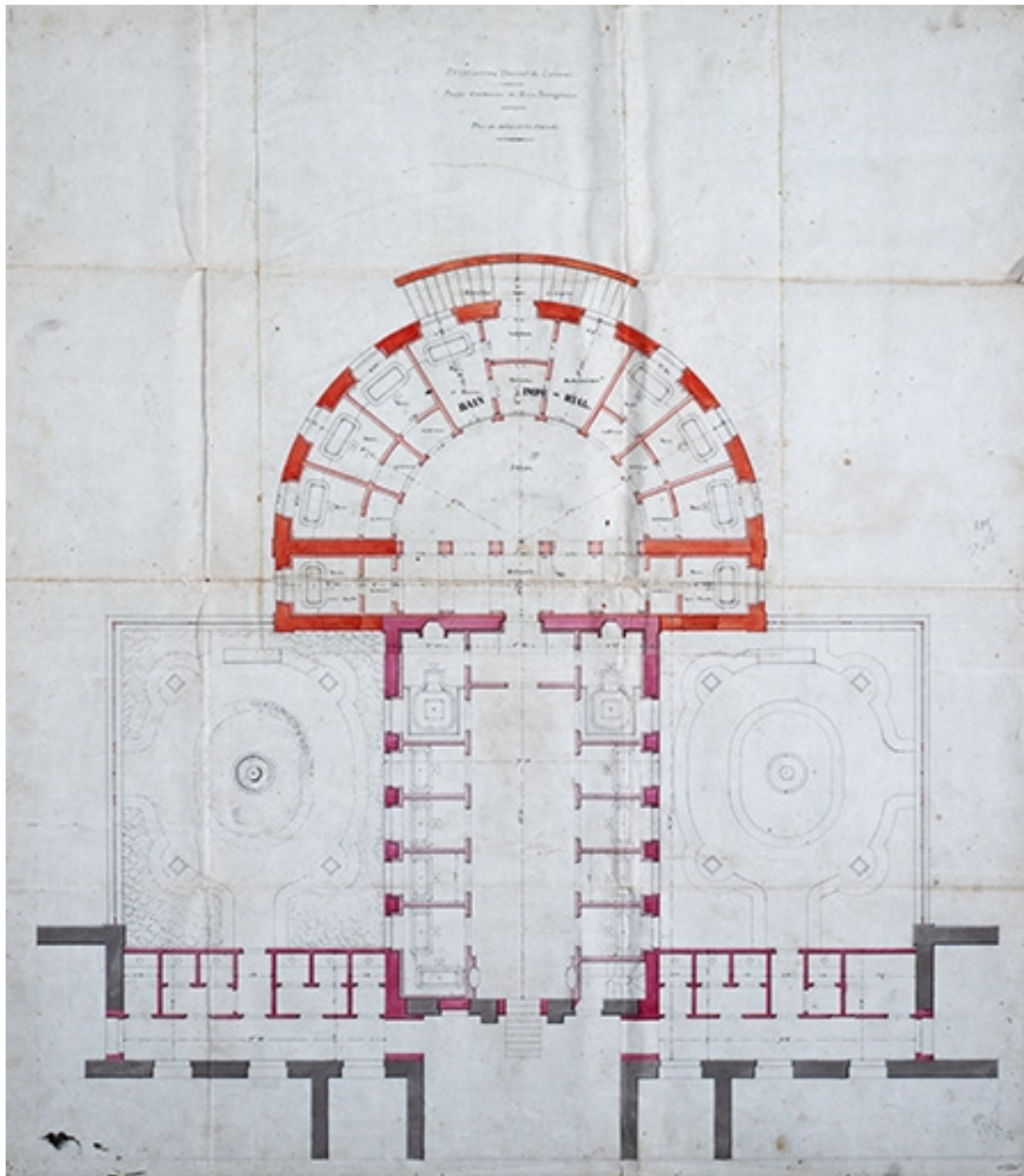
Projet de Bain impérial ferrugineux, plan du rez-de-chaussée (vers 1857).
