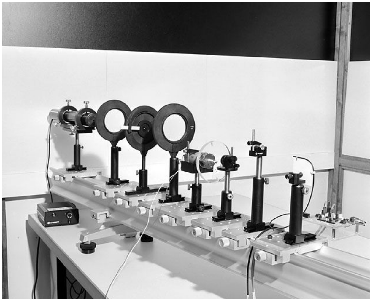
Banc d'optique. Bâtiment de l'enseignement (F), Optique instrumentale (salle F011).
