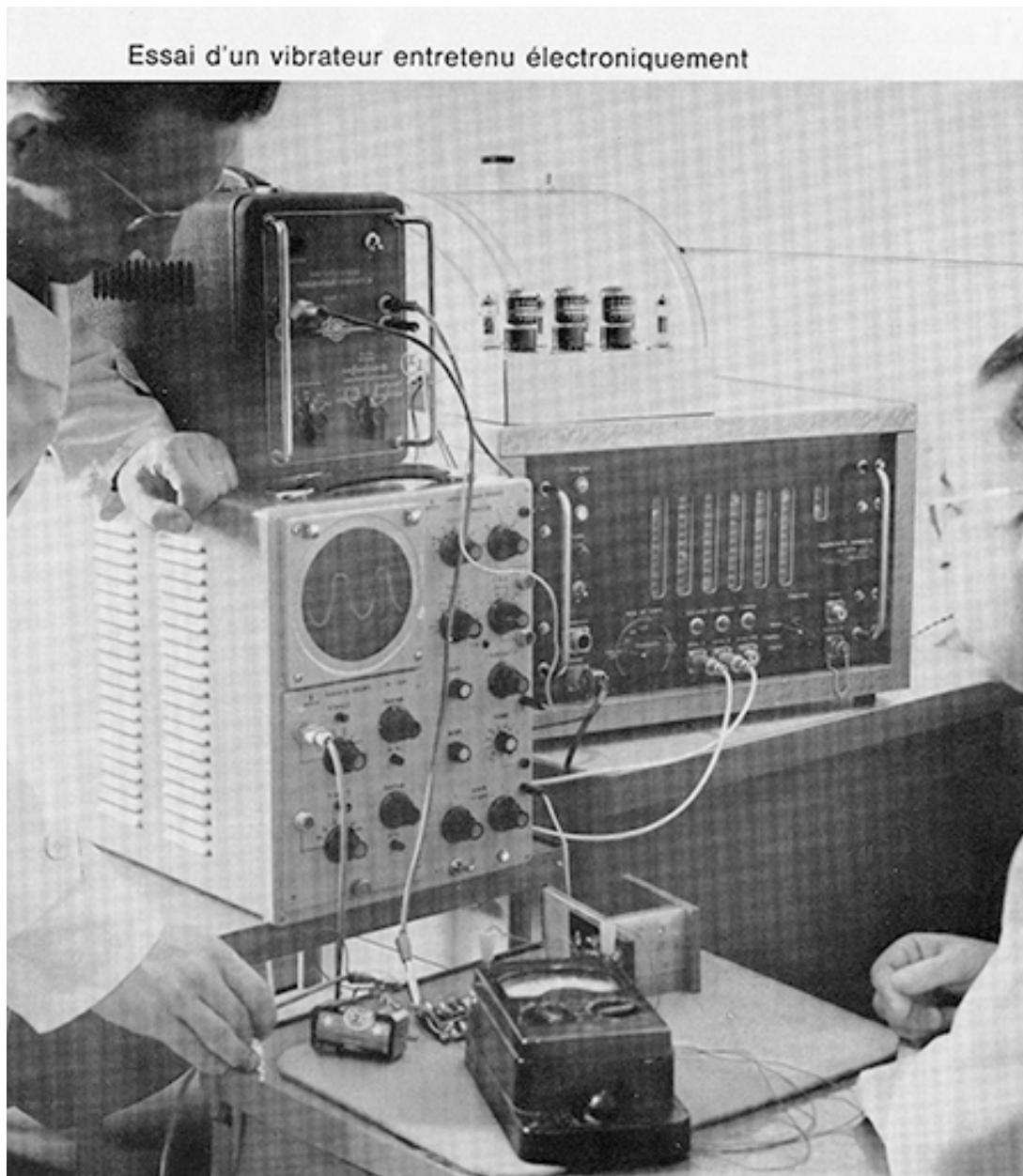
Essai d'un vibreur entretenu électroniquement, 1964.
