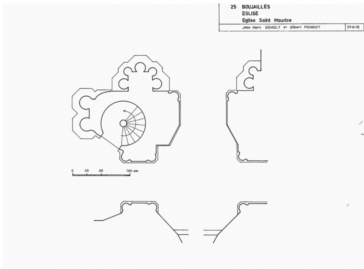
Plan des pilliers d'entrée : relevé-croquis J.M Demoly et G. Poinot, 1975.
