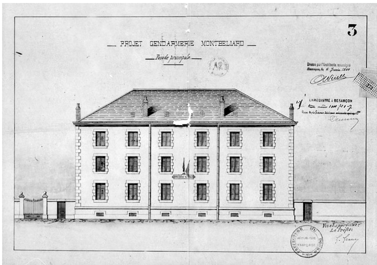
Projet de Gendarmerie à Montbéliard. Elévation de la façade principale, 1888.
