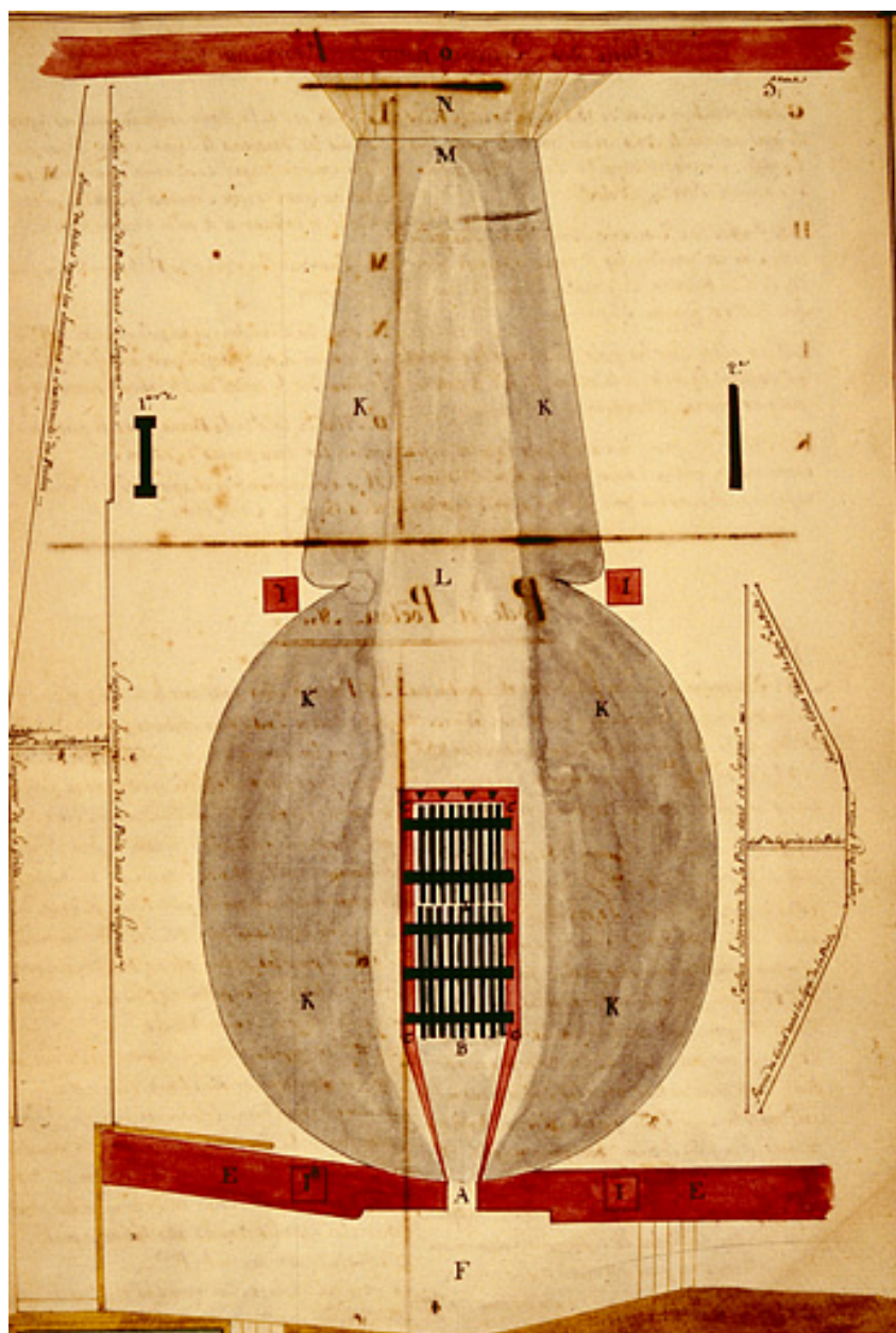
Fourneau et foyer d'une Poêle et d'un Poëlon, dessin, 1756.
