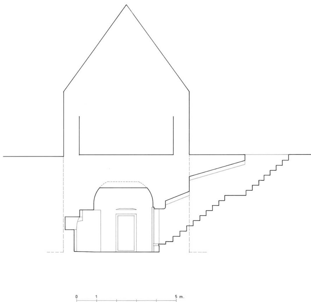
COUPE B-B'
