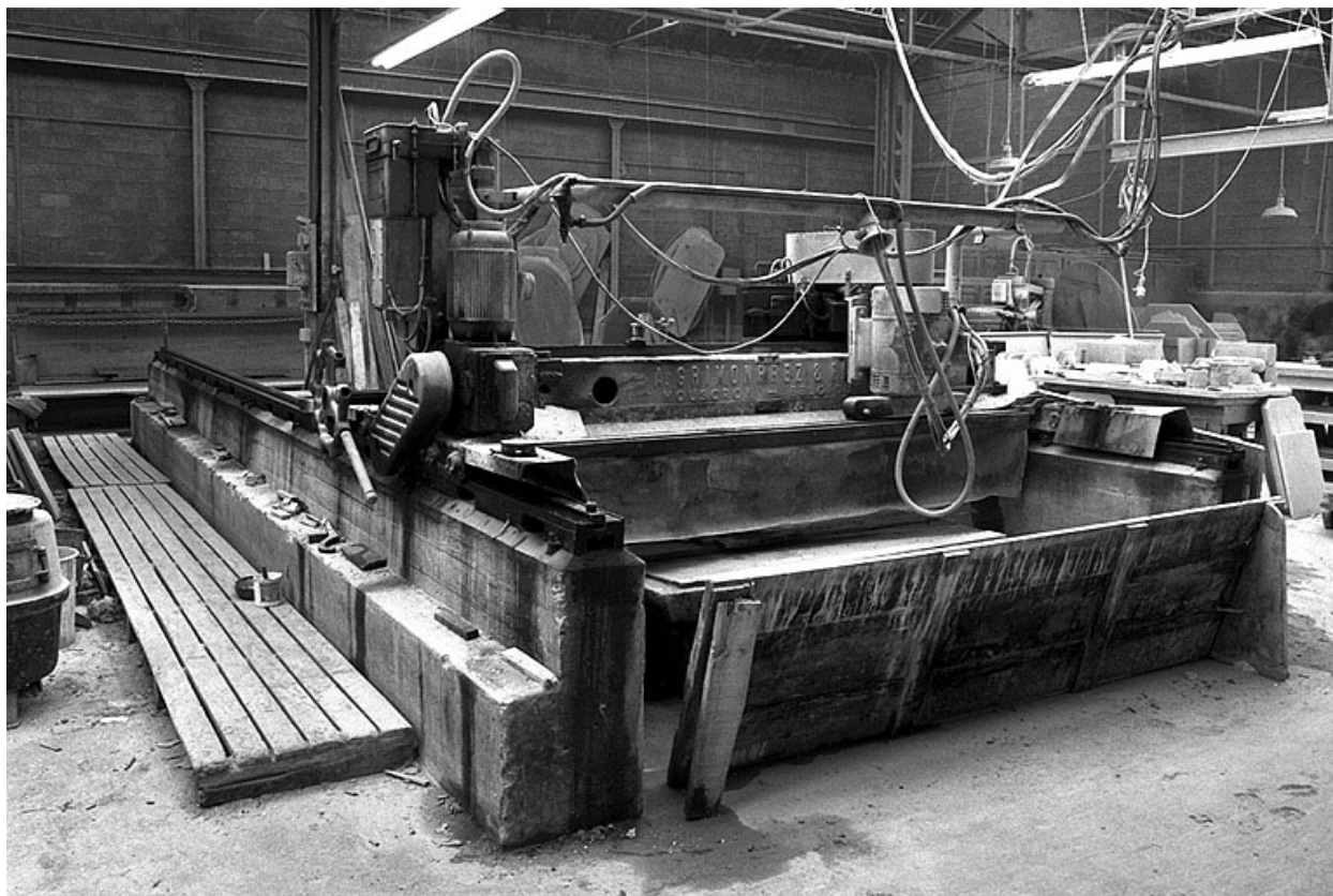
Usine de taille de matériaux de construction Célard, à Saint-Amour : l'un des deux polissoirs automatiques à plat.
