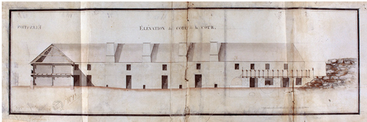
Elévation du côté de la cour.
