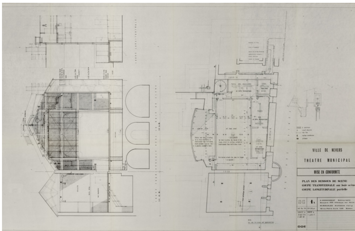
Ville de Nevers. Théâtre municipal. Mise en conformité. 1A. Plan des dessous de scène. Coupe transversale sur baie scène. Coupe longitudinale partielle. 1976.
