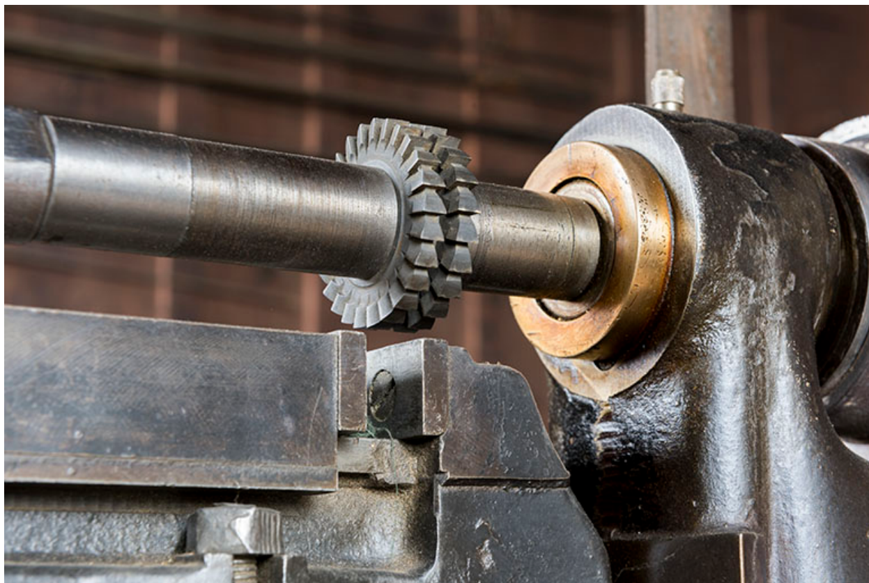
Détail des fraises.
