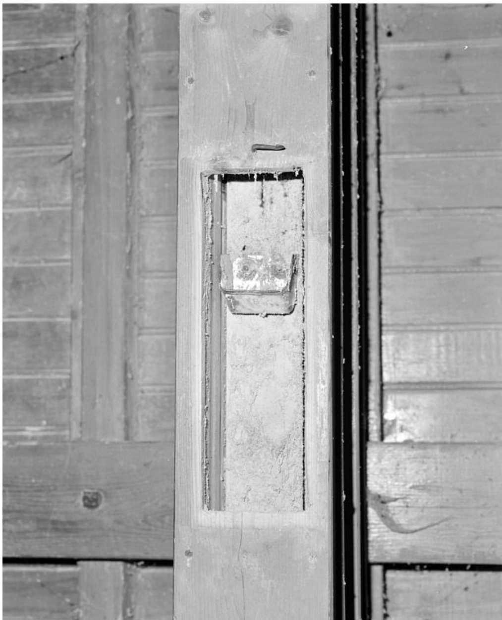
2e étage. Elévateur à godets, détail.
