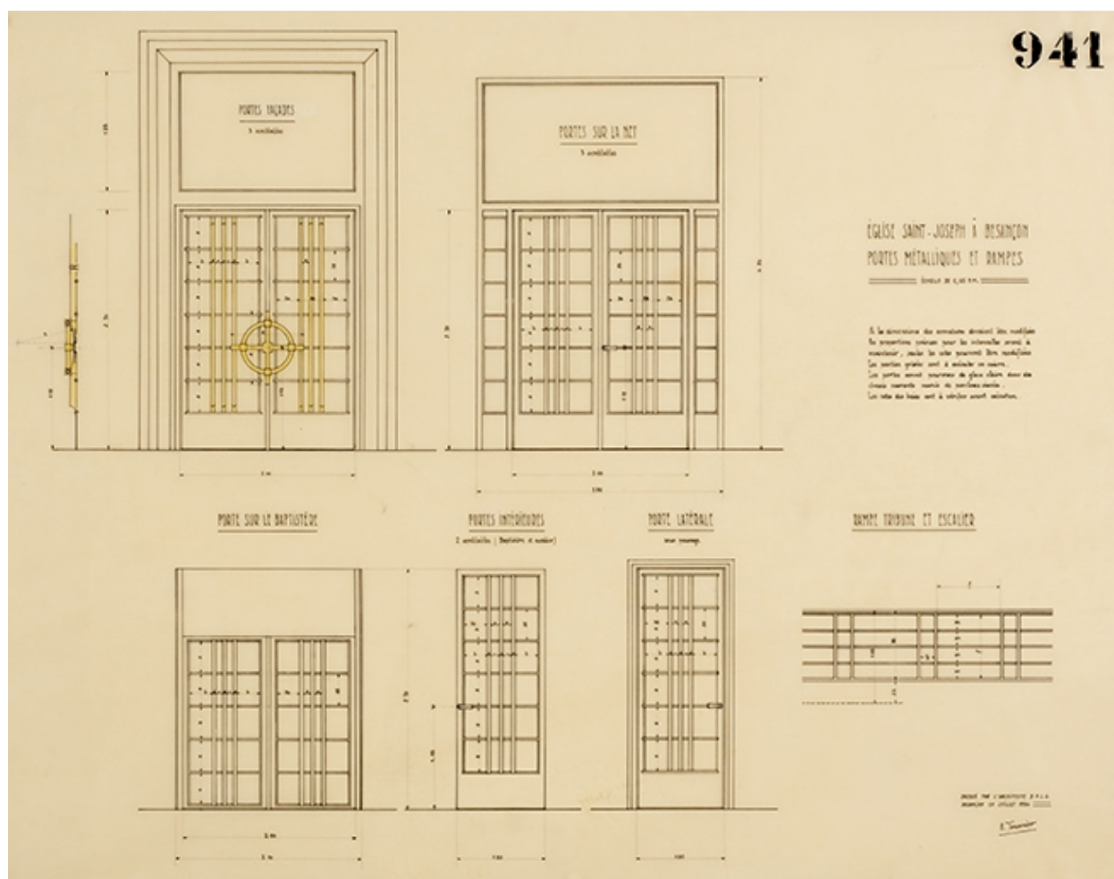
Dessin des portes de l'église Saint-Joseph à Besançon. Juillet 1954.
