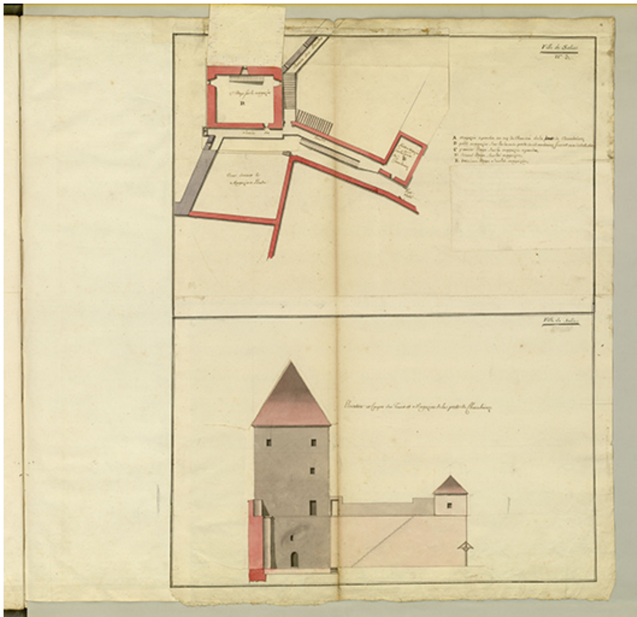
Folio 14. Ville de Salins. Tour et magasin à poudre de la porte de Chamboinoz. N°3. Plan, coupe et élévation. Deuxième étage sur le magasin, 1756.
