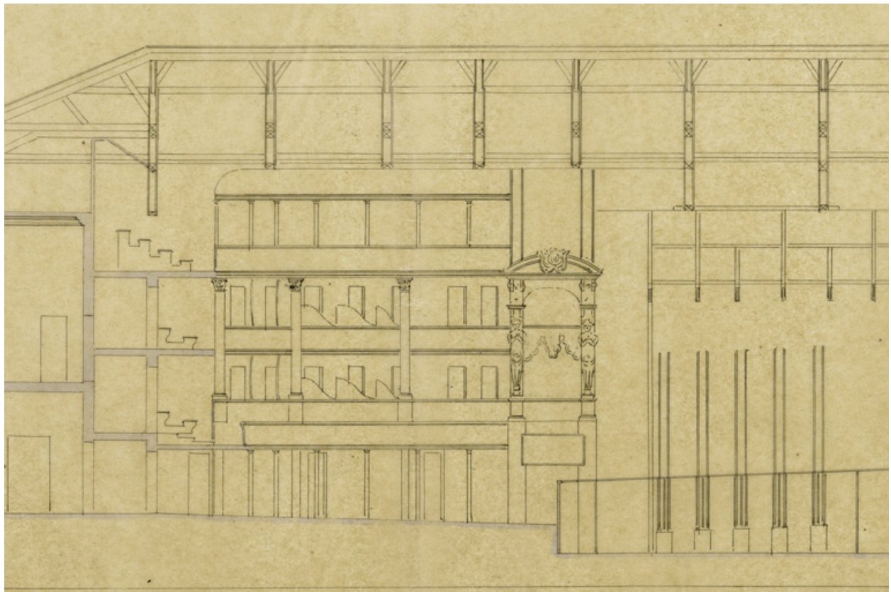
Projet de restauration de la salle de spectacle de la ville de Nevers. Coupe longitudinale [détail de la salle]. 9 avril 1851.
