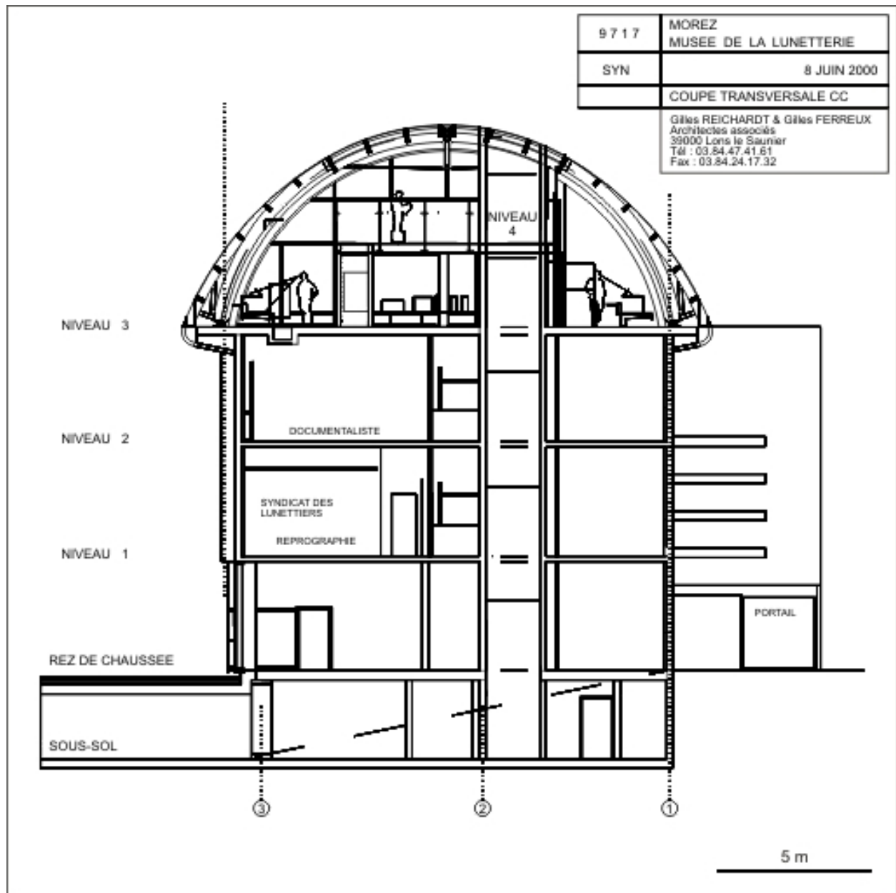
Coupe transversale CC, 2000.
