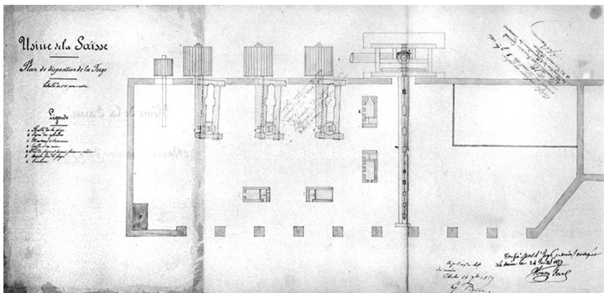
Usine de la Saisse. Plan de disposition de la forge [...].
