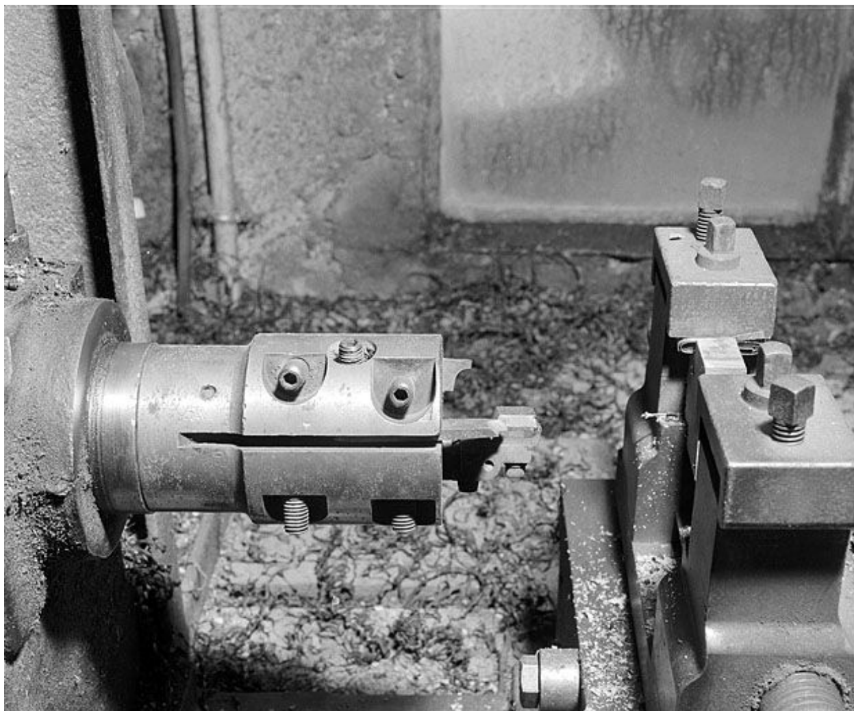
Détail du mandrin porte-outils.
