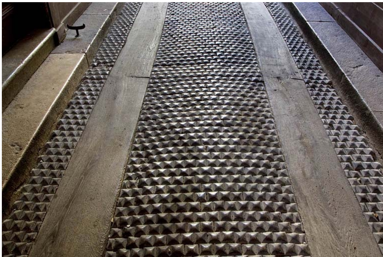
Deuxième logis secondaire, passage cocher : détail des pointes de diamant en bois constituant le sol.
