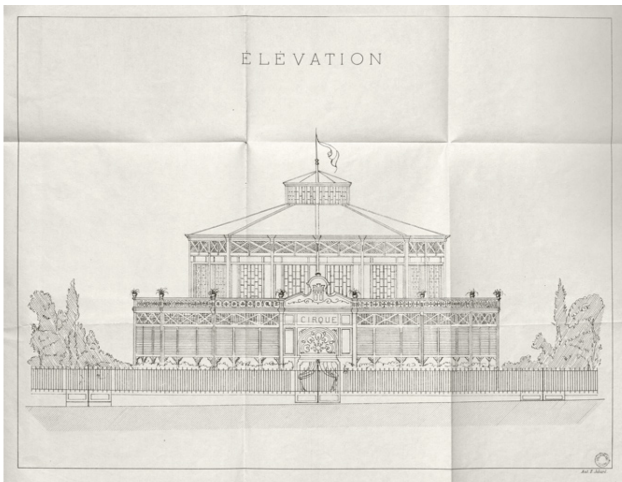
Cirque de Dijon [Cirque-Théâtre d'Eté, 4 cours du Général de Gaulle]. Elévation. S.d. [1869].
