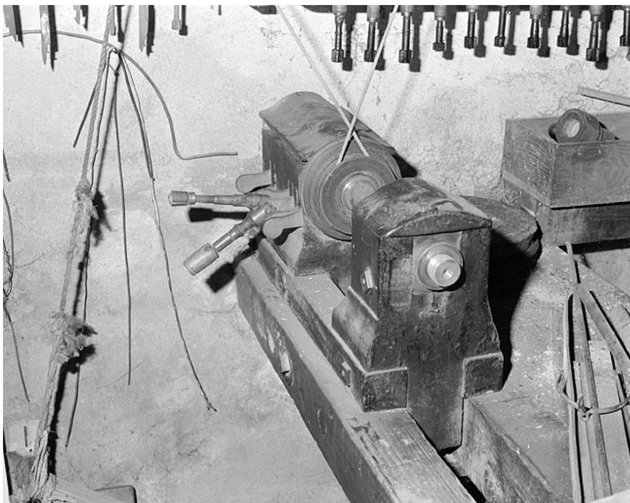
Tour à marchepied : clavier et clés de sélection.
