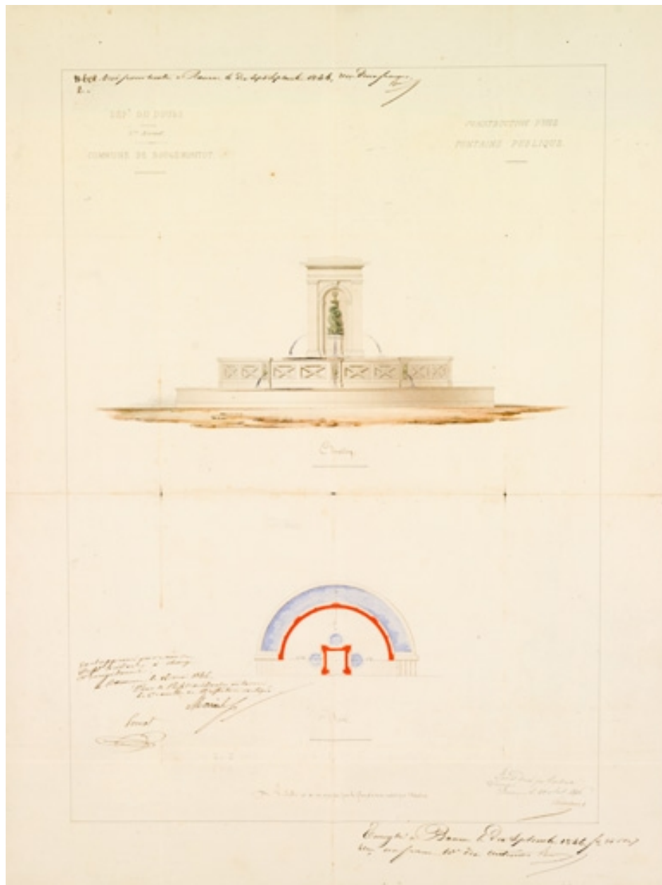
Construction d'une fontaine publique. Elévation. Plan. 1846.
