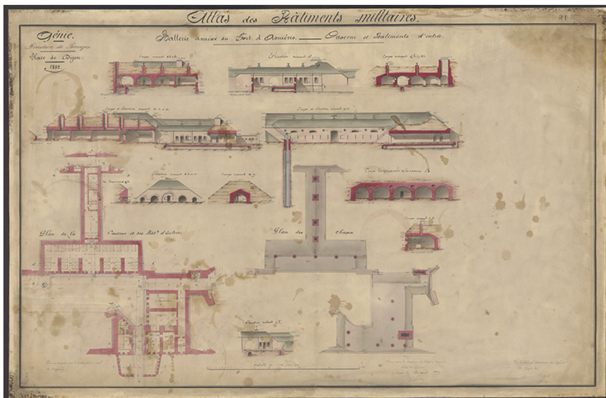
Batterie annexe du Fort d'Asnières - Caserne et bâtiments d'entrée. 1882 [signé par le chef du Génie le 20 avril 1885].
