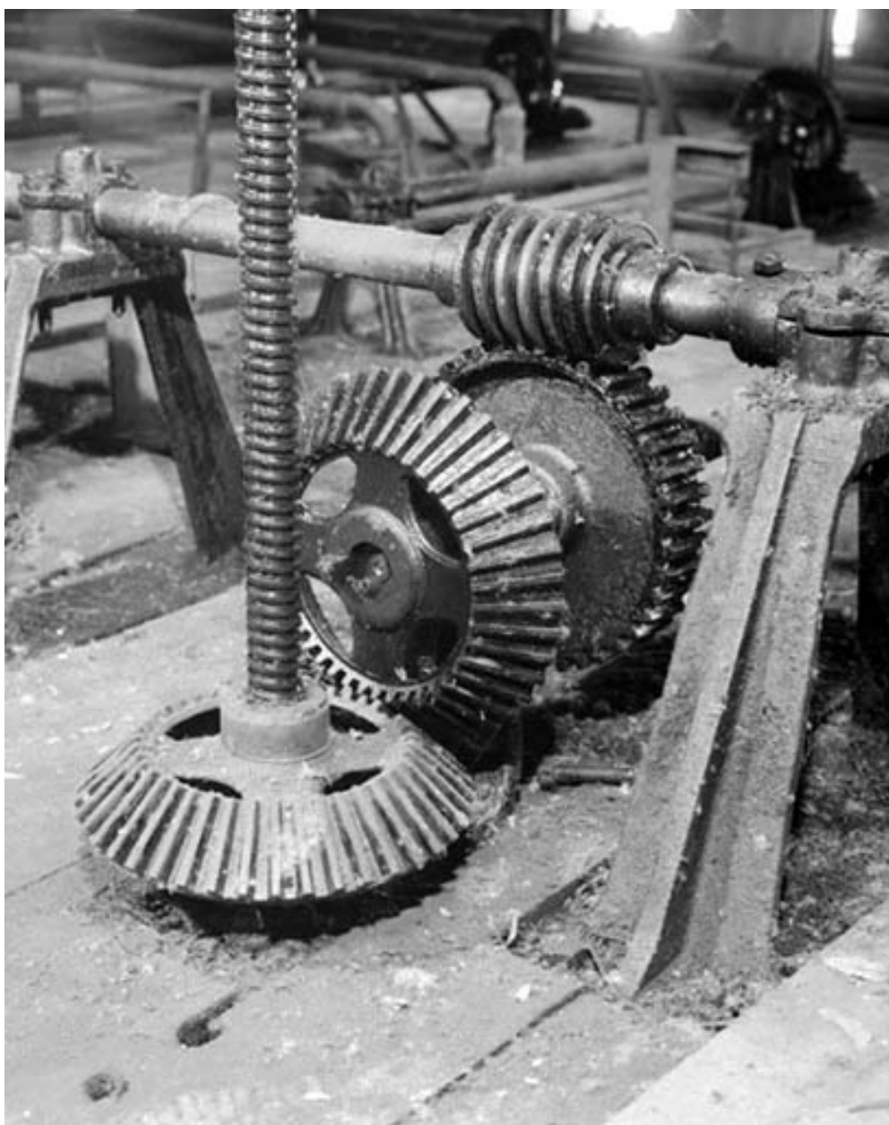
Système de descente à vis : détail.
