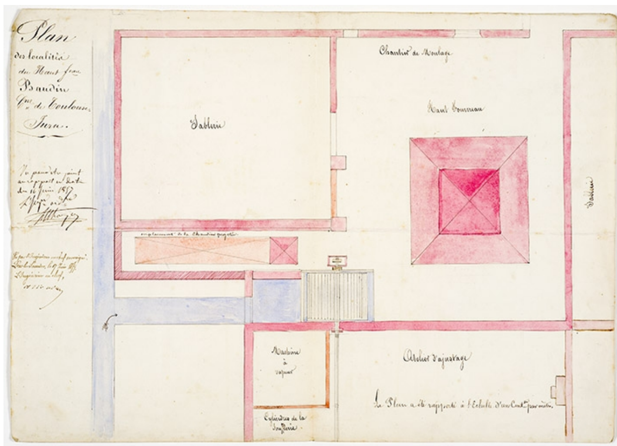
Plan de détail de la chaudière, plume, lavis, 1857.
