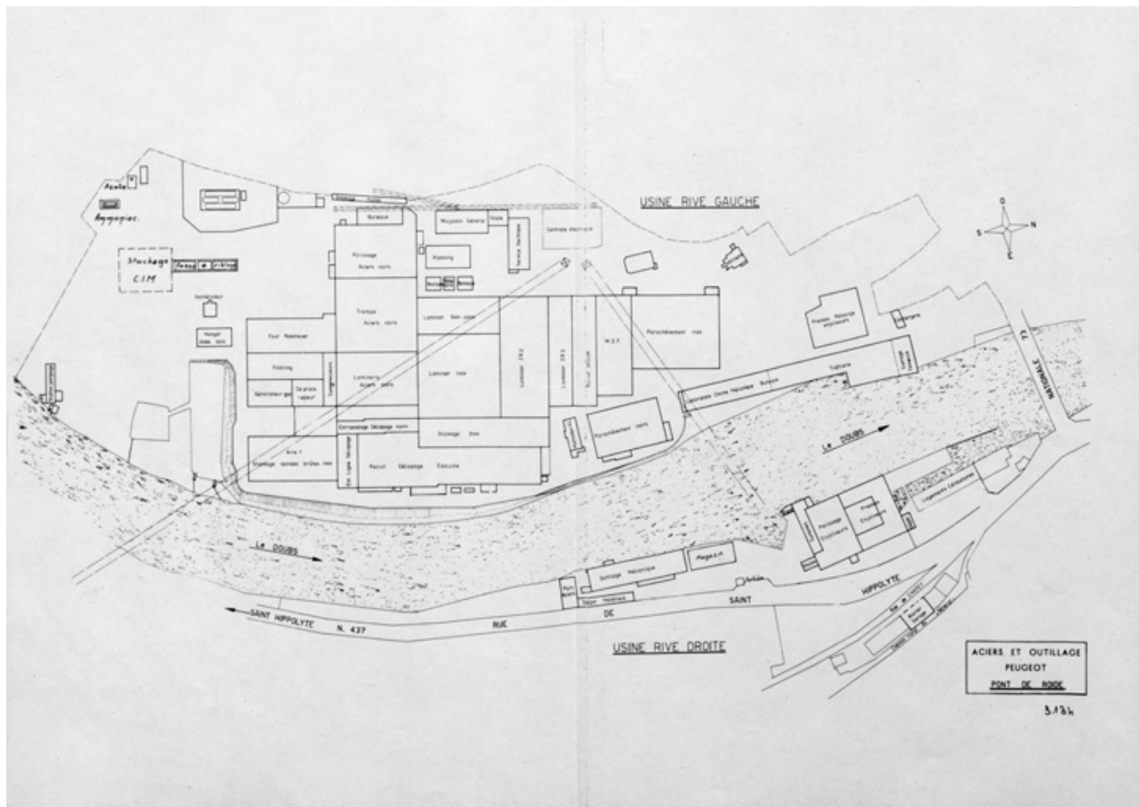
Plan-masse de l'usine AOP en 1970, tirage.
