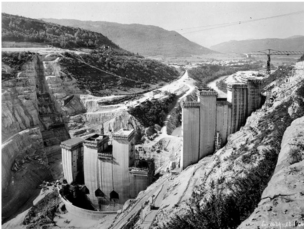
Barrage de Vouglans - Vue d'ensemble depuis amont rive gauche, 12 juillet 1966.
