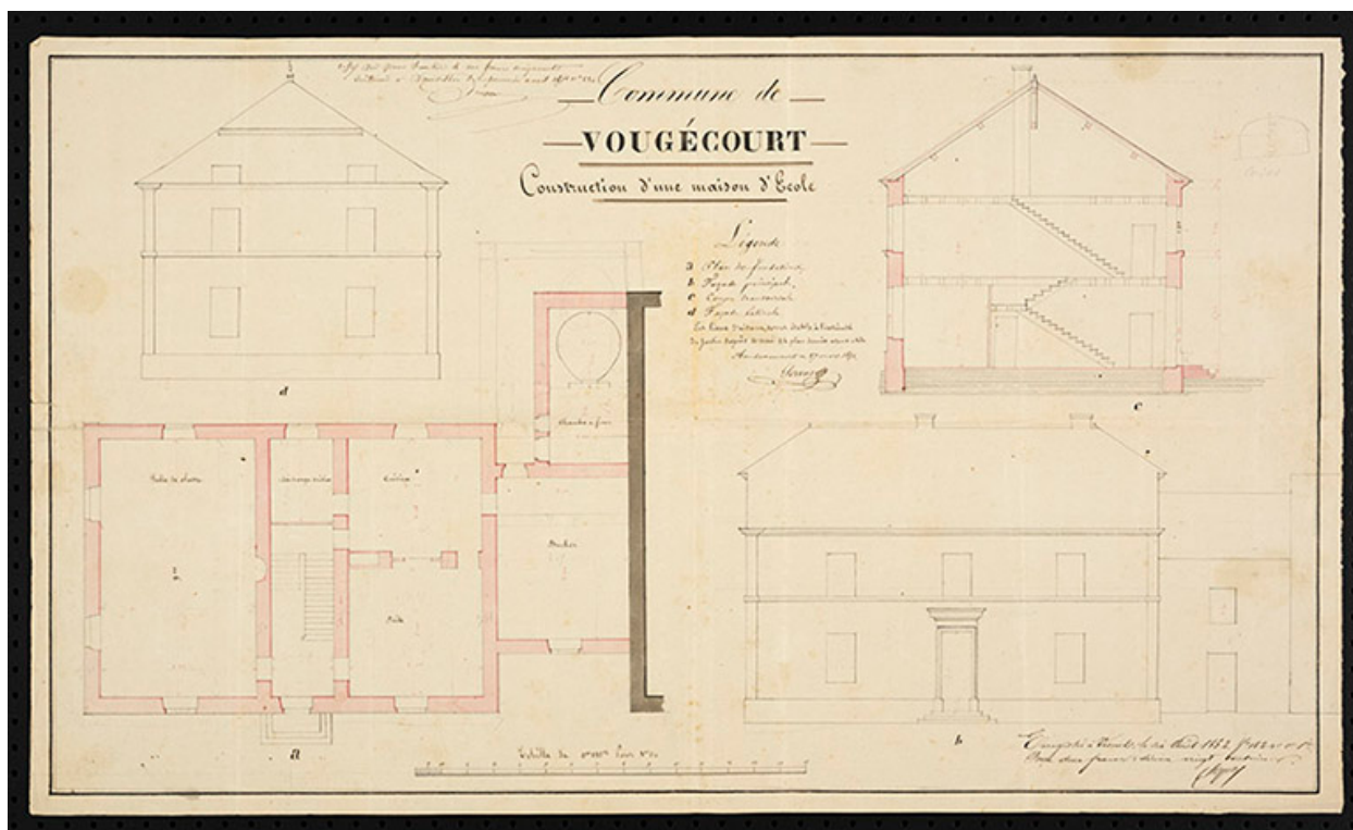
Construction d'une maison d'école et mairie. [plan, coupes et élévations] 1852
