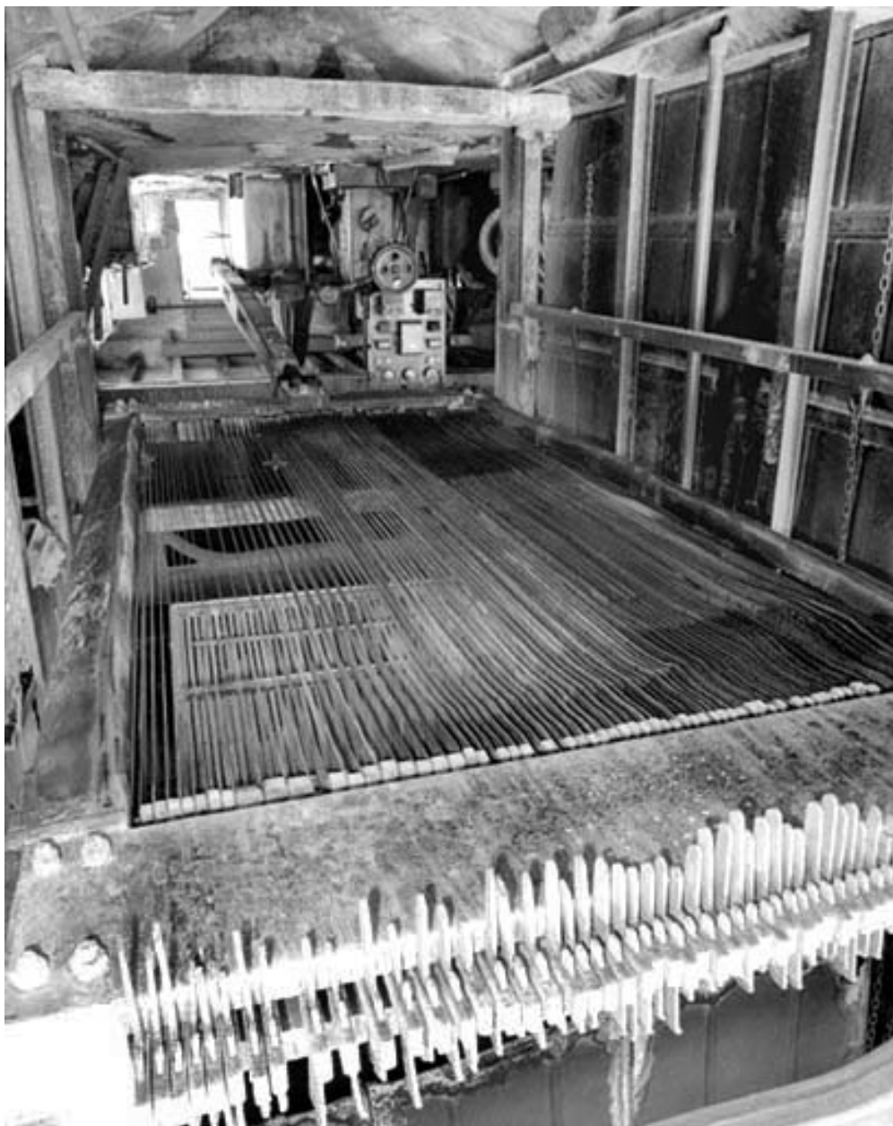
Châssis porte-lames.
