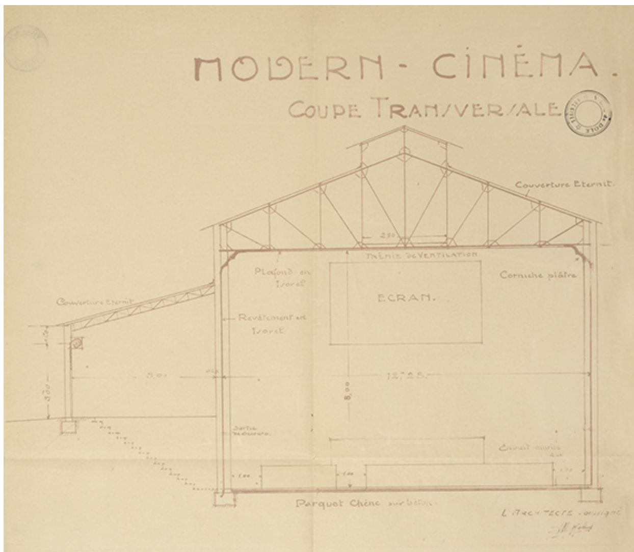
Modern-Cinéma. Coupe transversale. S.d. [1936].
