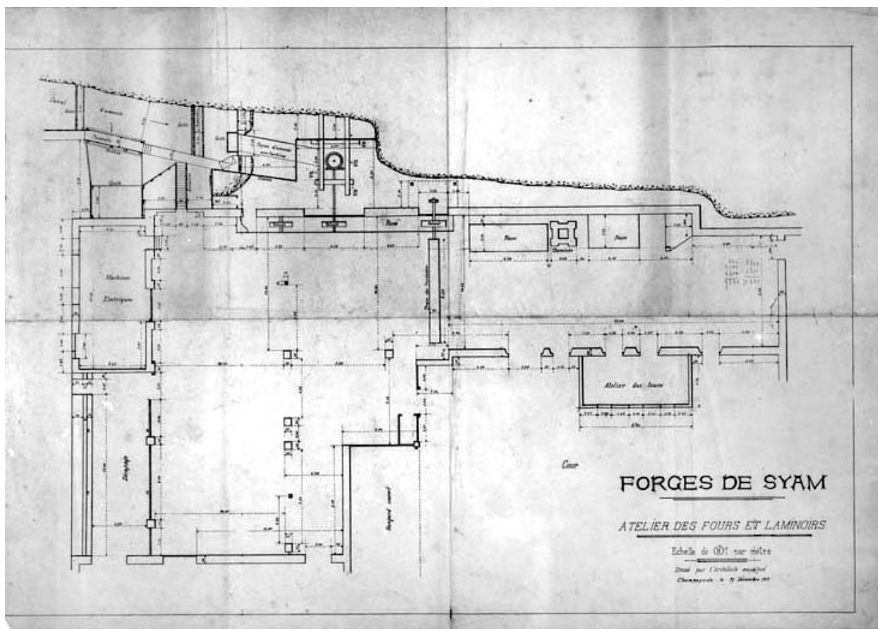
Forges de Syam. Atelier des fours et laminoirs.
