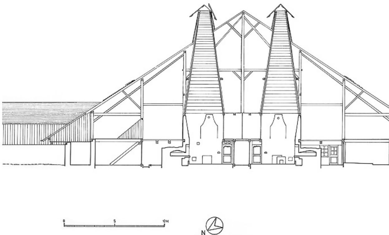
Coupe transversale.
