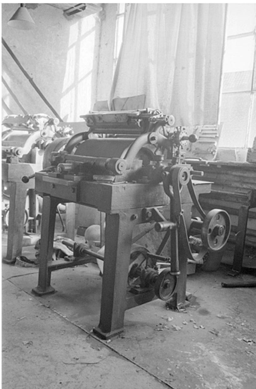
Appareil à cylindre. Porte-pierres baissé.
