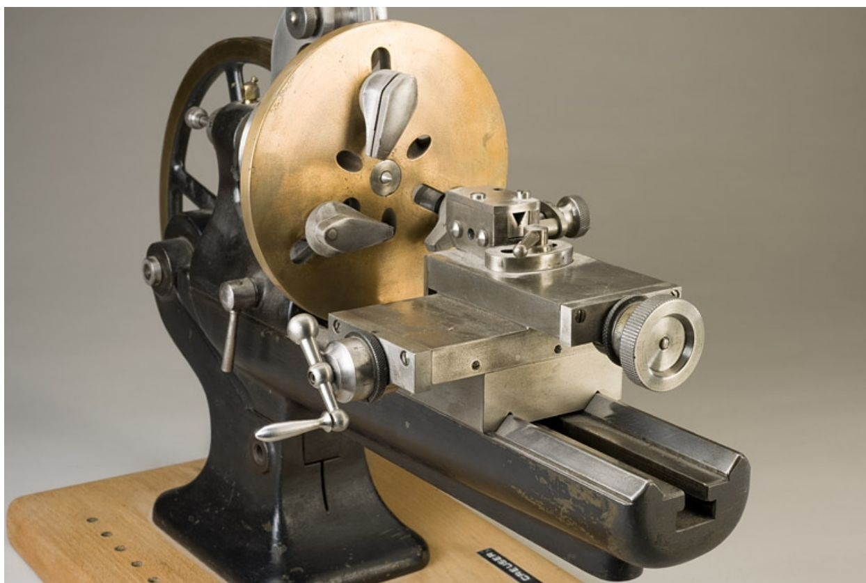
Perche, chariot porte-outil et porte-pièce, vu de trois quarts.
