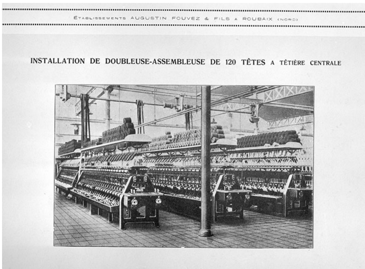
Installation de doubleuse-assembleuse de 120 têtes à têtère centrale.
