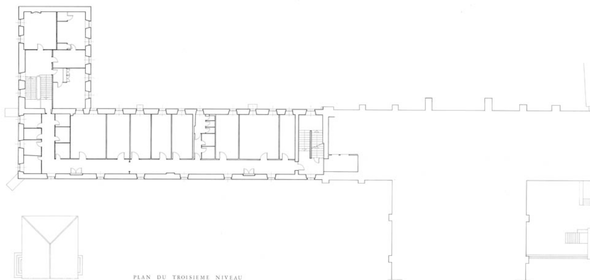
plan du troisième niveau
