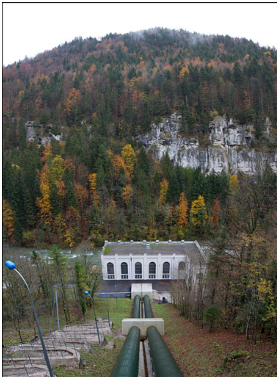
Centrale hydroélectrique du Refrain, Charquemont.
