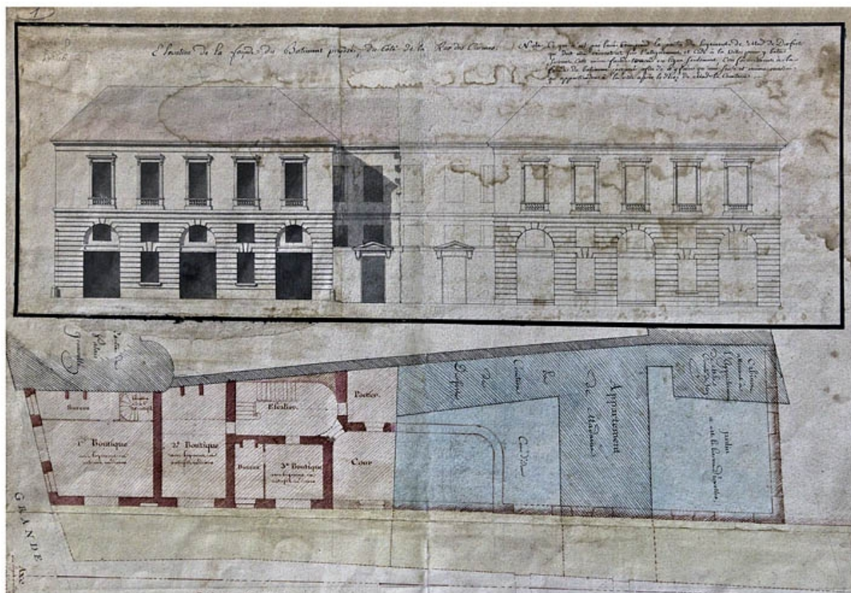
Plan de l'élargissement de la ruelle des Carmes : détail de l'aménagement contre le palais Granvelle. Dessin, plume et aquarelle, 24 mars 1783.
