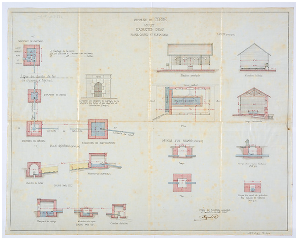
Commune de Corre. Projet d'adduction d'eau. [plans, coupes, élévations.] 1910
