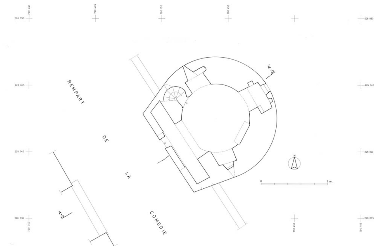
Tour Blondeau : plan du niveau supérieur.
