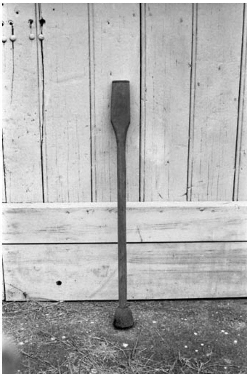
Fouloir de mouleur à main.
