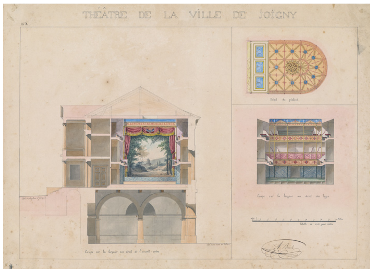
Coupe sur la largeur au droit de l'avant-scène, Coupe sur la largeur au droit des loges [et] Détail du plafond. N° 8. S.d. [1829-1830]. (MAP : G/82/89/2008-039064)
