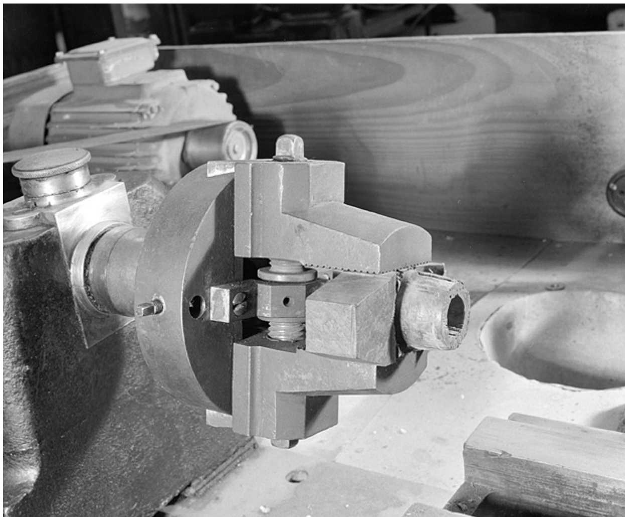
Mandrin "gueule de loup" (atelier principal).
