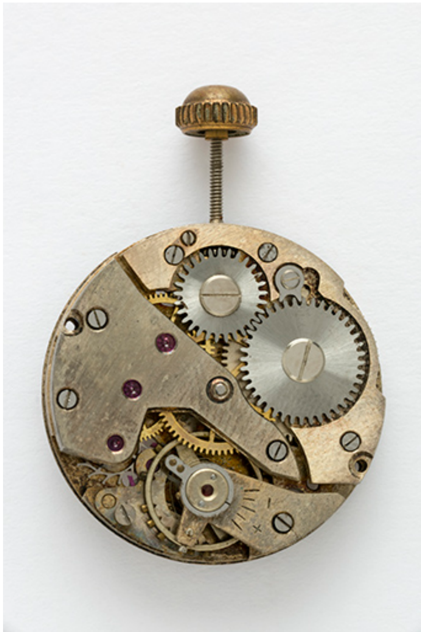
Mouvement de montre mécanique Cupillard VC 233, à Villers-le-Lac, 1ère moitié 20e siècle.
