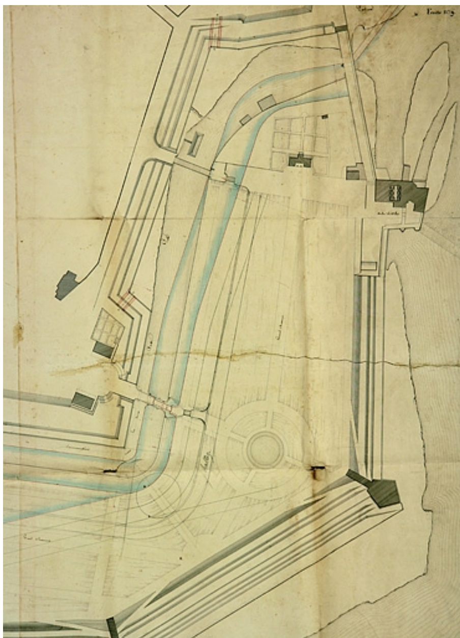
Plan général des ouvrages proposés dans la dérivation de Chamars [détail : partie aval], 1824.
