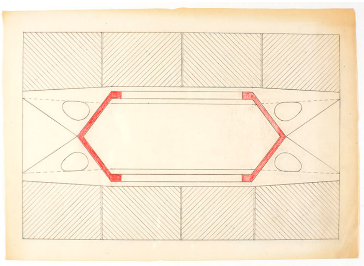
Dessin du coffrage de la base (pile) montrant la sous-face du premier étage, André Maisonnier, s.d.
