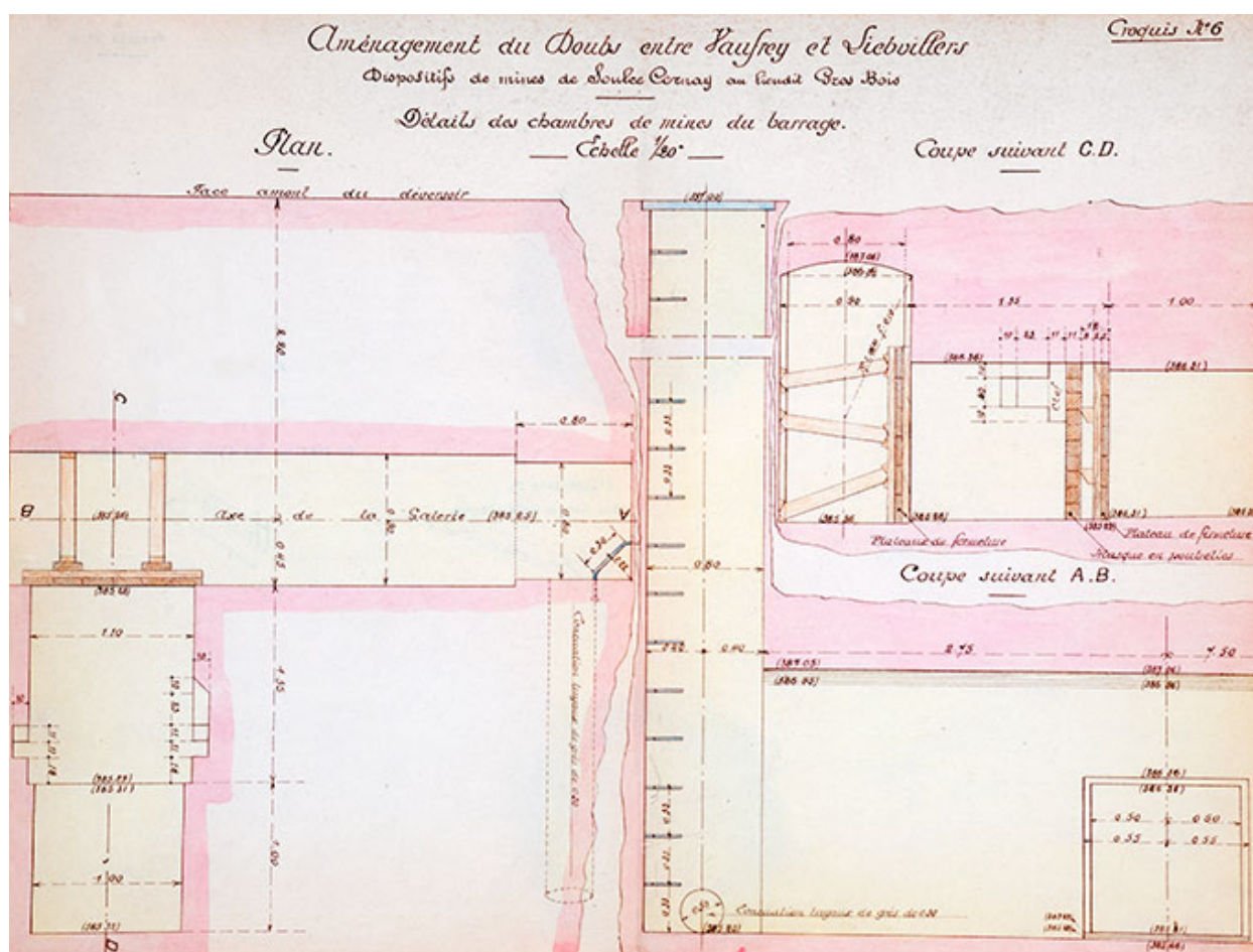
Aménagement du Doubs entre Vaufrey et Liebvillers. Dispositifs de mines de Soudce Cernay au lieu dit Gros Bois. Croquis n° 6. Détails des chambres de mines du barrage [plan et coupe], 1924.
